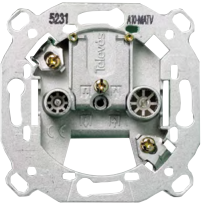
Toma TV-FM Derivación única (Fabricante TELEVÉS)
