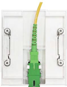
Vista interior con la fibra óptica montada
