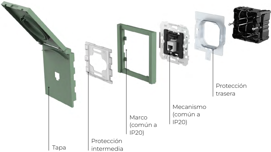
Explosionado Cosmos RJ IP44:
