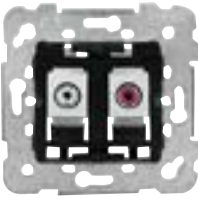
Toma estéreo RCA 18576 Emborne trasero rápido por perforación de aislante. Cable: máximo 3 pares de 0,3 mm²
