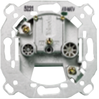
Toma TV-FM Serie 2-10 Final serie Derivación única (Fabricante TELEVÉS)
