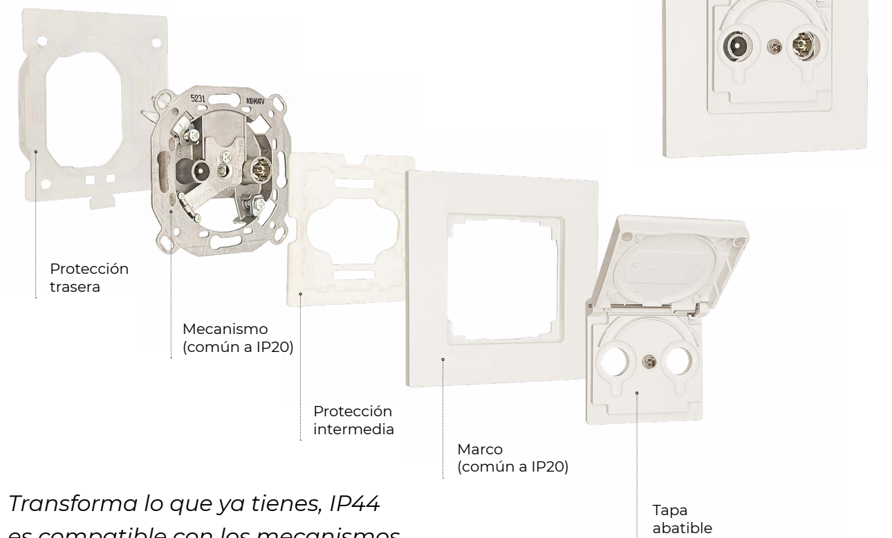
Ejemplo de montaje Miro TV IP44
