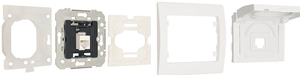
Ejemplo del Iris RJ IP44
